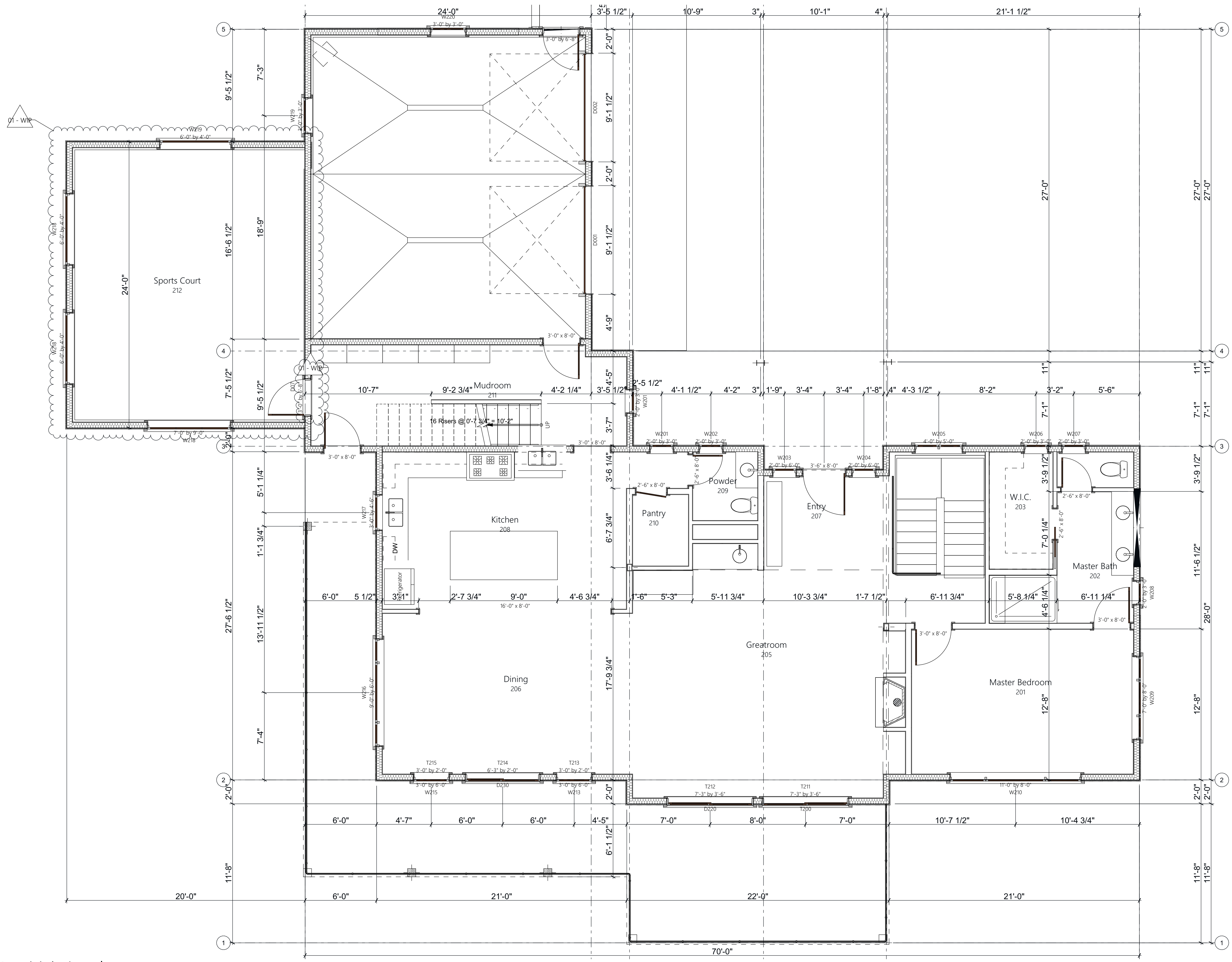
1 Main Level SCALE: 1/4" = 1'-0"
